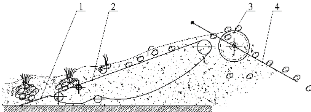
Рис. 1.8. Схема картоплекопача КБН-2Б:
