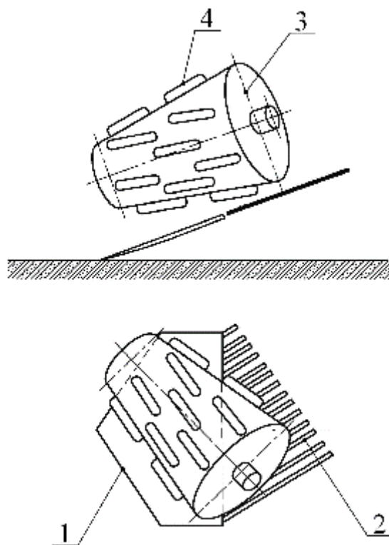
Рис. 1.3. Схема картоплекопача:
