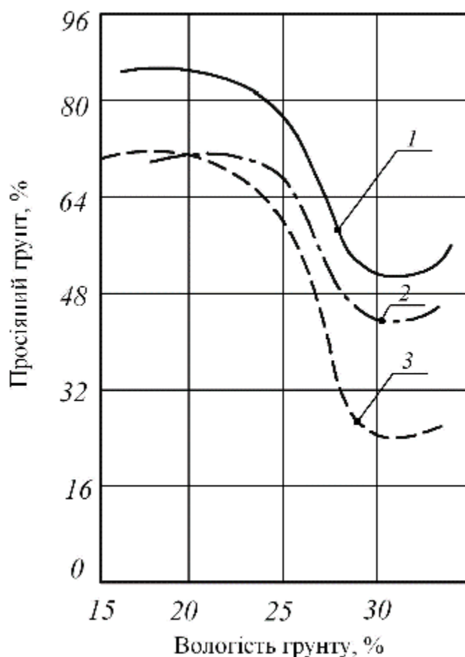
Рис. 1.1. Залежність просіювання ґрунту (важкий суглинок) від вологості:
