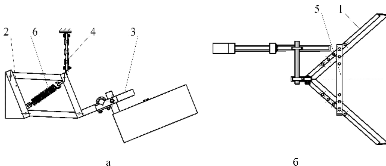
Рис. 2.3 Схема розподільника:
