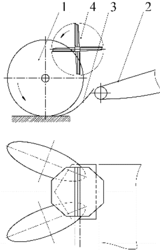
Рис. 1.5. Схема комбінованого підкопувального робочого органа:
