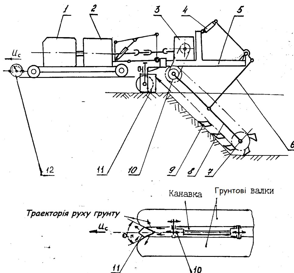
Рисунок 3.1 – Схема лабораторної установки (на проекції – вид в плані рама і привід умовно не показані): 1, 2, 3 – електропривод з варіатором, 4-регульована по довжині ланка, 5 – рама, 6 – поводок, 7, 10 – зірочки ланцюгового контуру, 8 – рамка контуру, 9 – скребок, 11 – подільник-відбивач, 12 – динамометр
