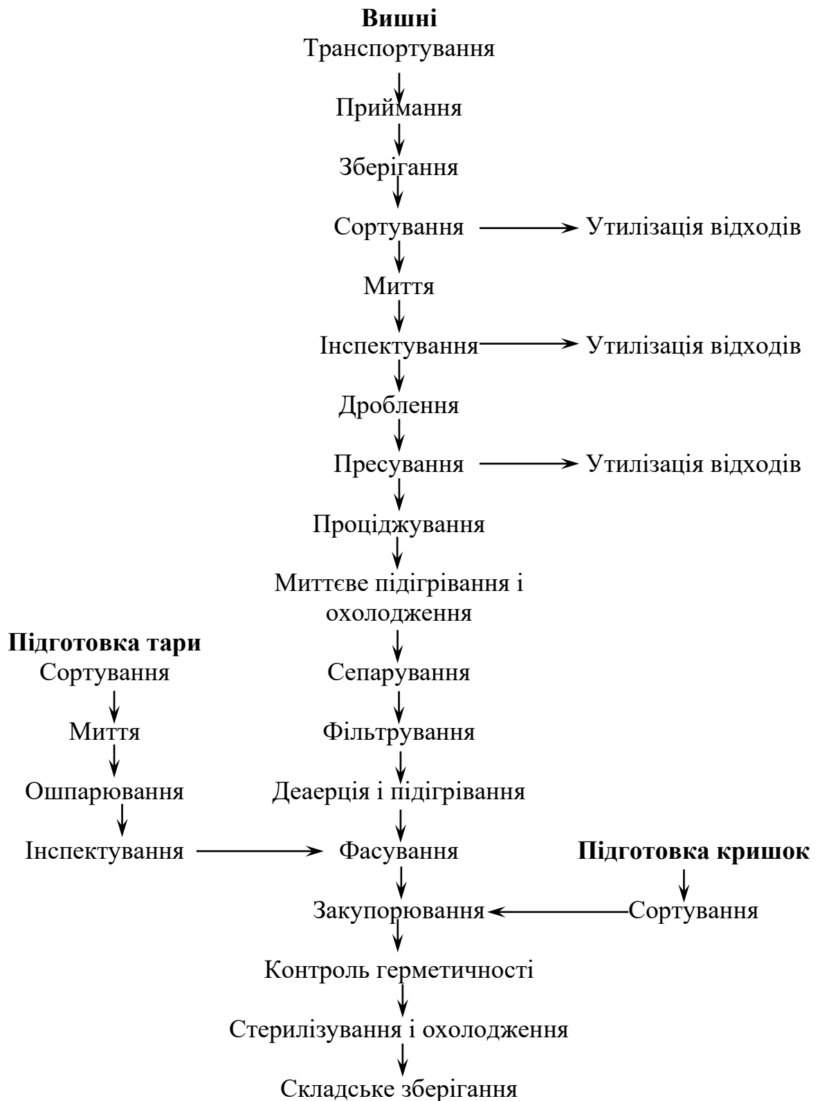
Рис 2.1. Технологічна схема виробництва консервів «Сік вишневий натуральний»
