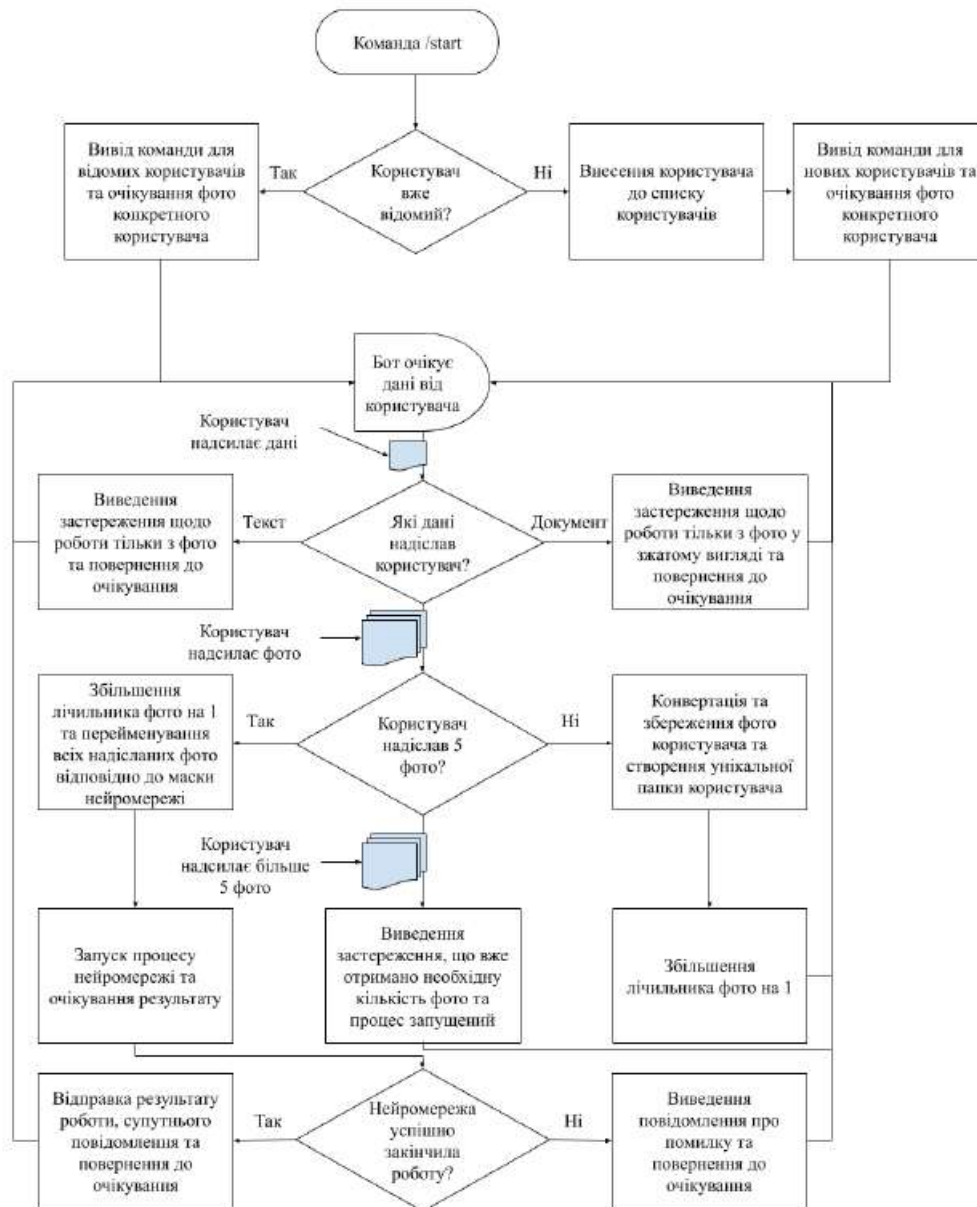
Рис. 3.17 Блок-схема роботи Telegram-боту з нейронною мережею
