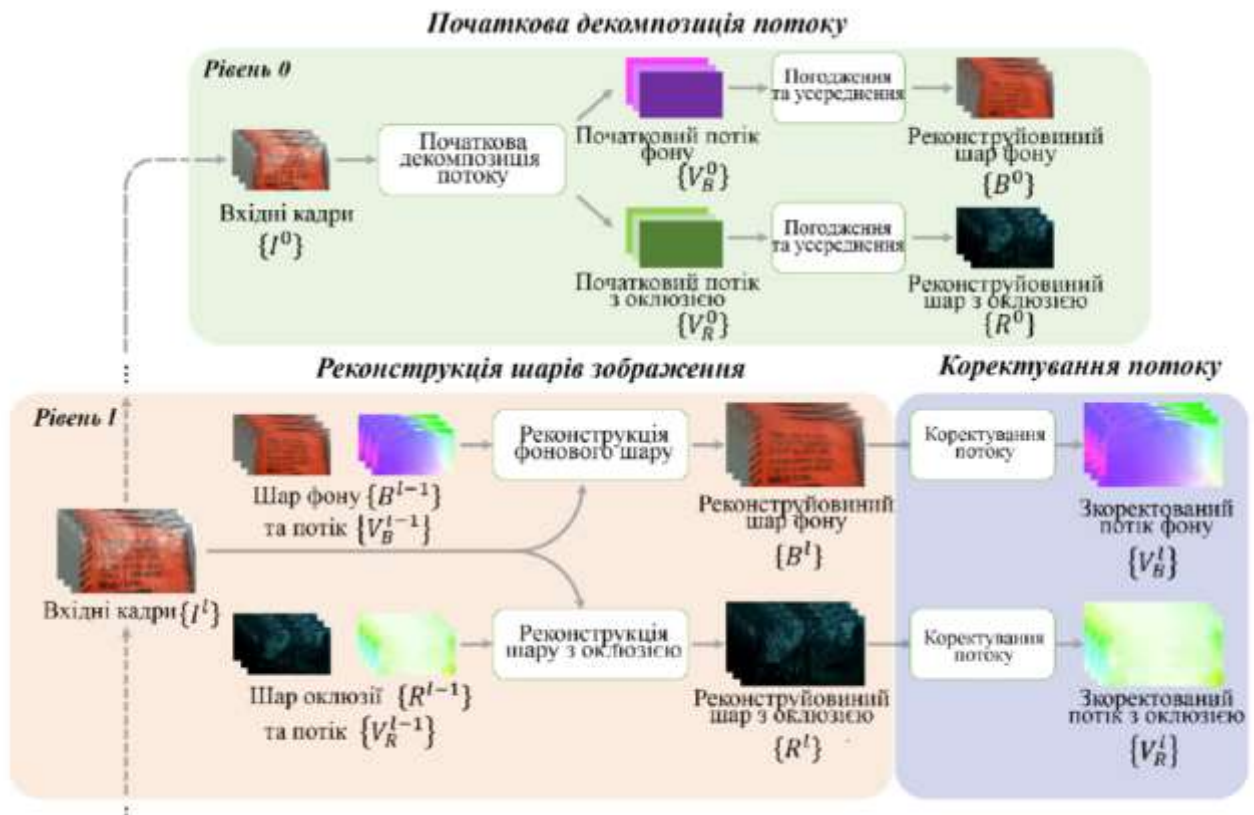
Рис. 2.1 Огляд алгоритму
