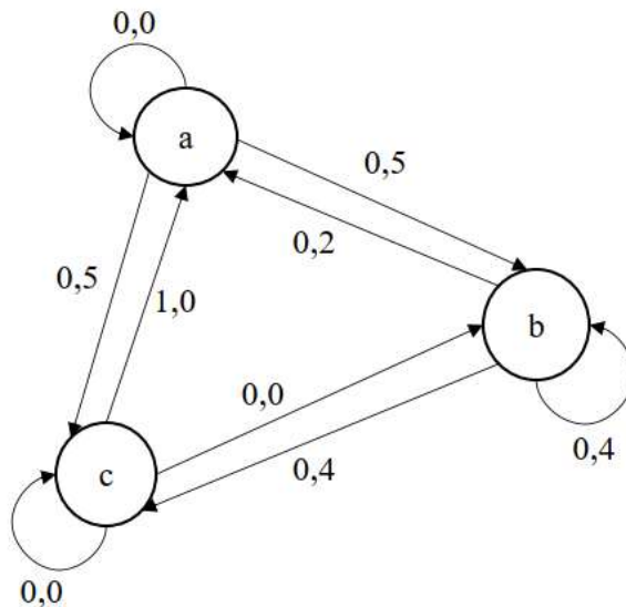
Рисунок 3.5 – Марківська модель першого порядку
