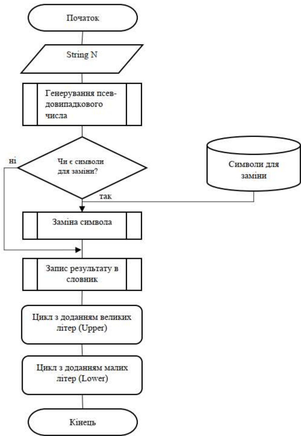
Рисунок 3.1 – Узагальнений алгоритм роботи програми
