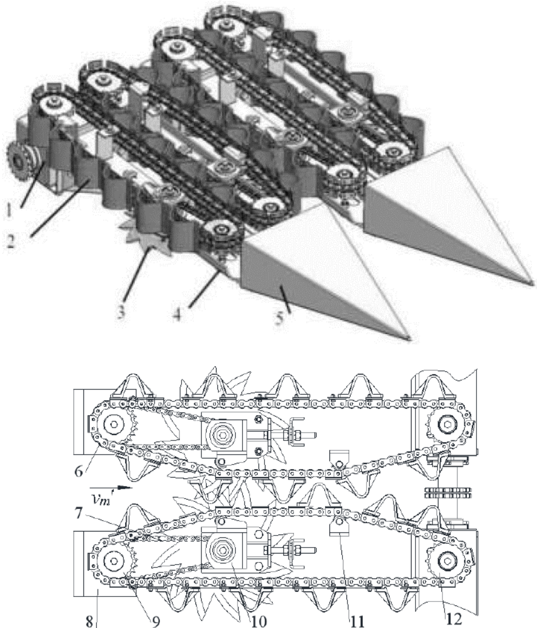
Рисунок 2.2. Затискно-транспортувальний пристрій. 1 – коробка передач, 2 – затискний елемент, 3 – ніж, 4 – опорна плита, 5 – носок подільника, 6 – транспортний ланцюг, 7 – ланцюг приводу фрези. 8 – натяжний пристрій ланцюга, 9 – ведена зірочка, 10 – привідний ланцюг, 11 – направляючий механізм ланцюга, 12 – привідна зірочка.
