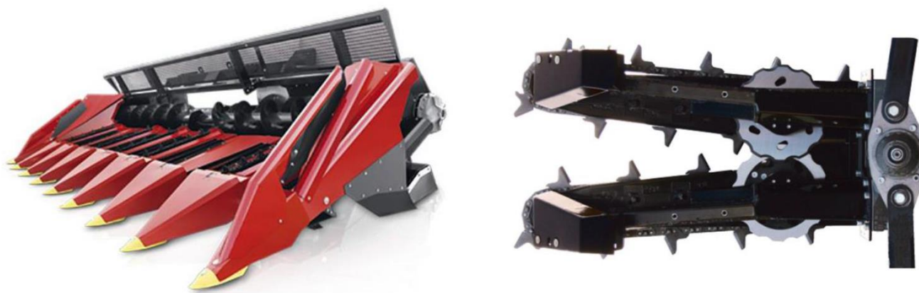
Рисунок 1.8. Соняшникова жатка Geringhoff SunStar.
