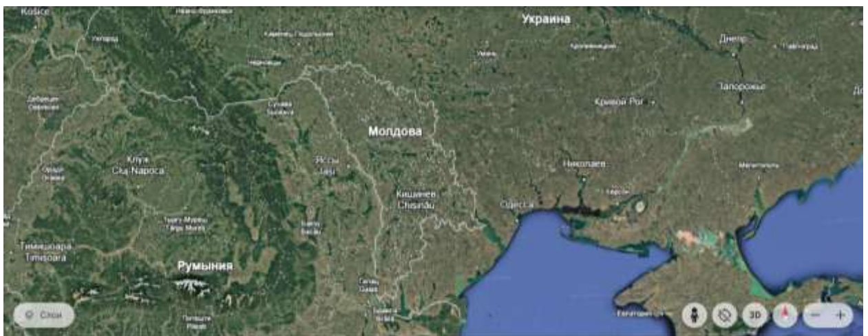
Рис. 2.3. Південні, західні та центральні території Правобережної України в програмі Google Earth (висота камери 903 км) [45]
