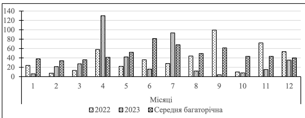
Рис. 2.2. Сума опадів за 2022-2023 рр., мм
