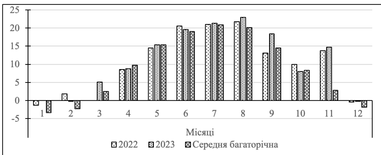
Рис. 2.1. Середньомісячна температура повітря за 2022-2023 рр., °C
