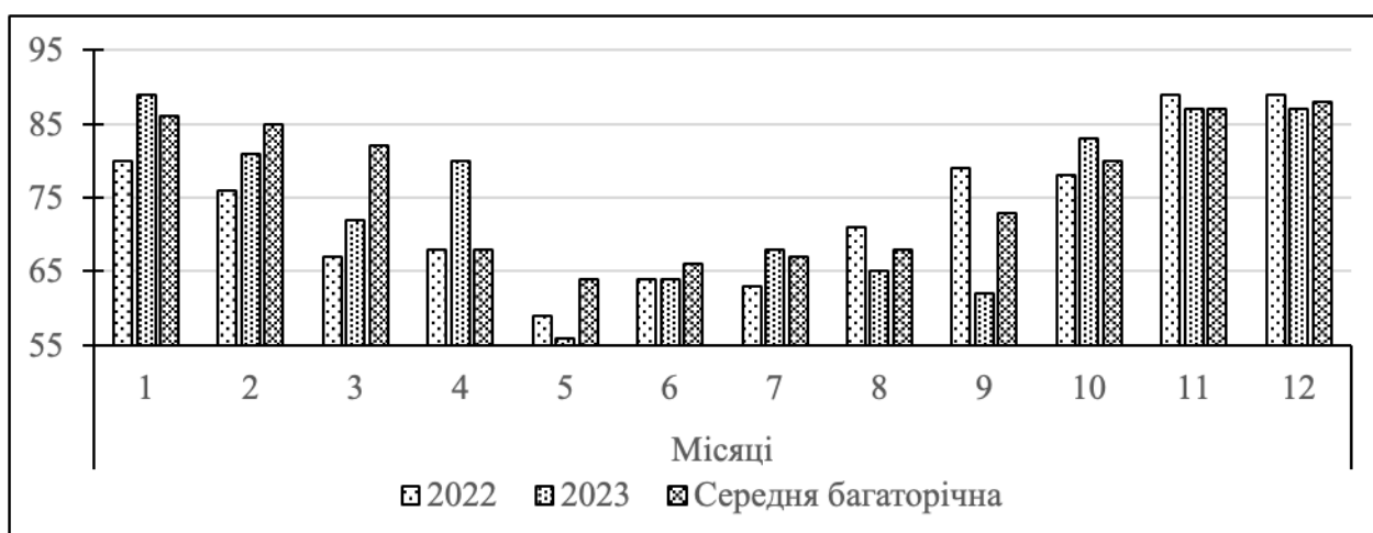
Рис. 2.3. Середньомісячна відносна вологість повітря за 2022-2023 рр., %
