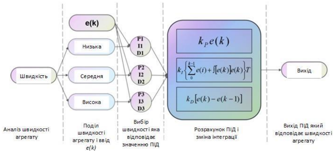
Рисунок 3.5 Принцип вдосконаленої структури алгоритму керування ПІД.
