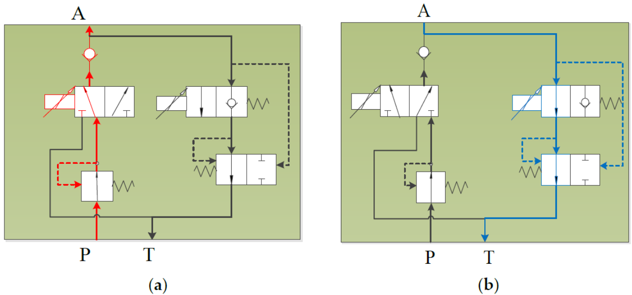
Рисунок 2.6 Принцип роботи інтегрованого електромагнітного пропорційного клапана. (a) підйом жатки; (b) опусканням жатки.
