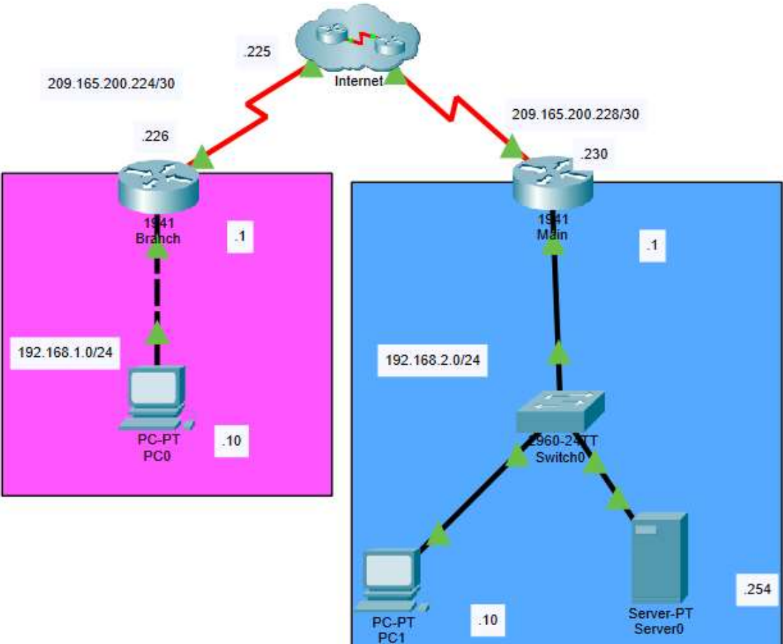
Рисунок 3.2- Топологія проектованої мережі.
