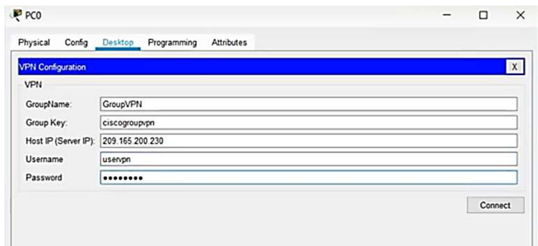
Рисунок 3.6- Під'єднання користувача VPN
