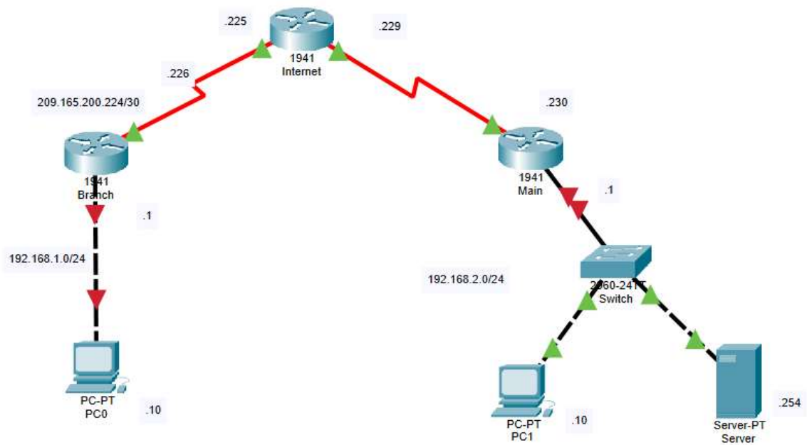
Рисунок 3.1 - Топологія проєктованої мережі.
