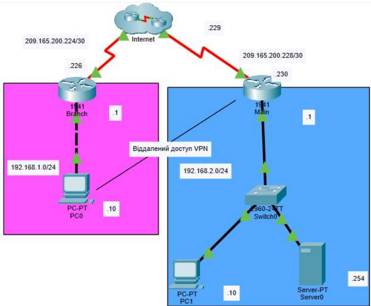
Рисунок 3.7- Спрощена топологія проєктованої мережі
