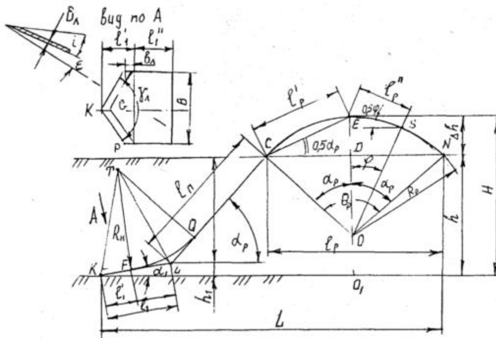
Рисунок 2.2 – До визначення параметрів профілю робочої поверхні
