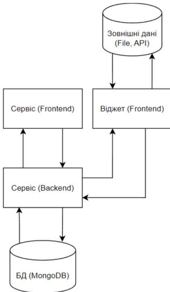
Рис. 3.1 Схема структури компонентів додатку та їх взаємодії
