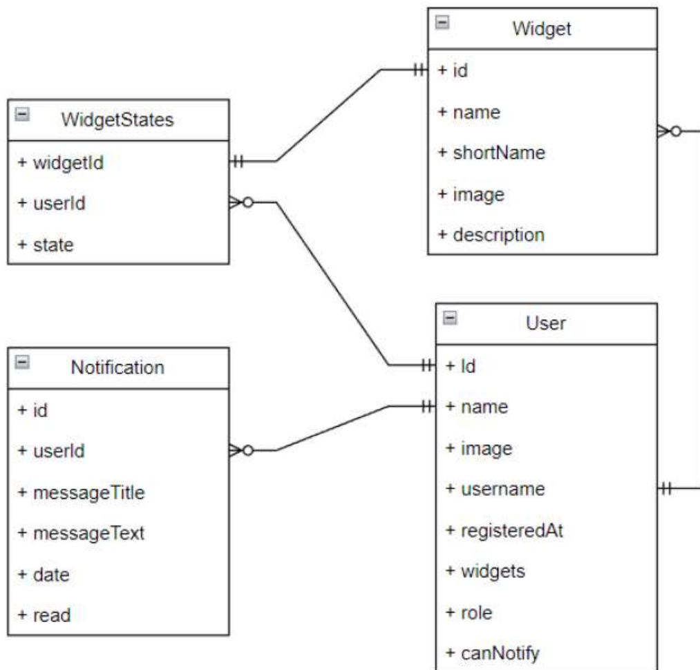
Рис. 3.2 ERD діаграма додатку
